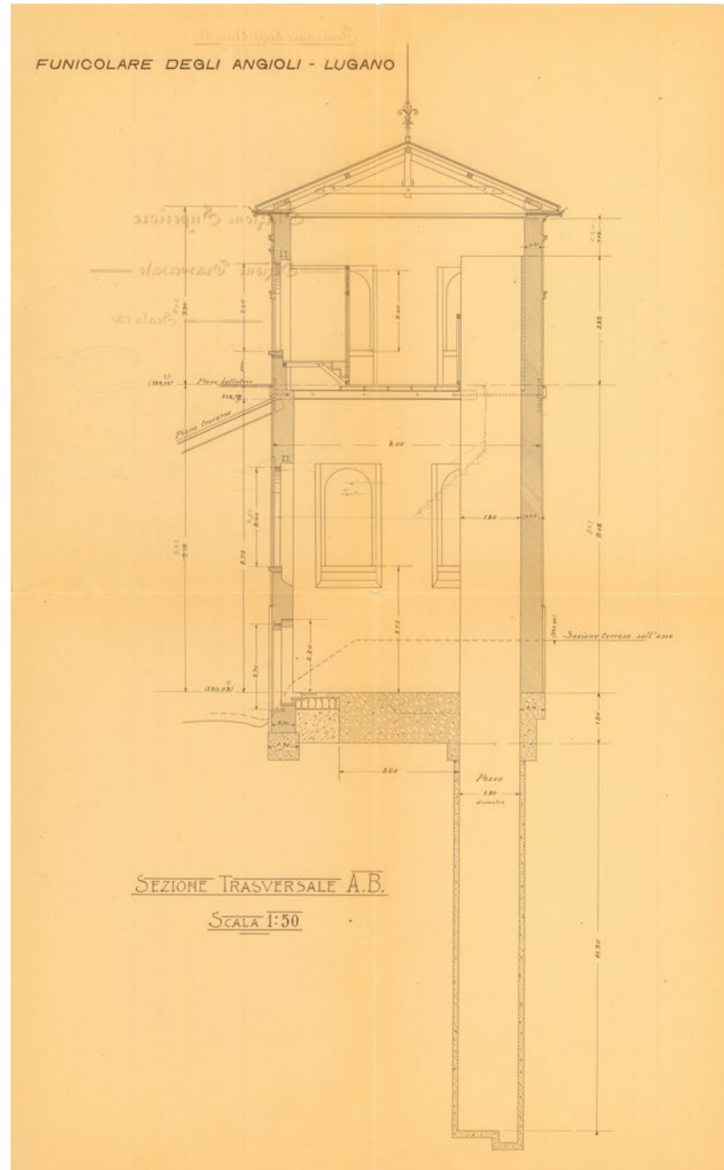
Vista e sezione della stazione a monte: torretta con pozzo per contrappeso; Piani originali 1911. La trazione viene attivata con un contrappeso che scorre nella fossa con dislivello di 21 m (rapporto 1:7).
